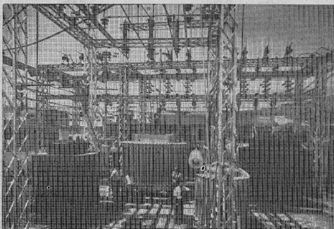
Instalando tres nuevos transformadores de 3750 KVA. cada uno, en la Subestación de Hatillo.
